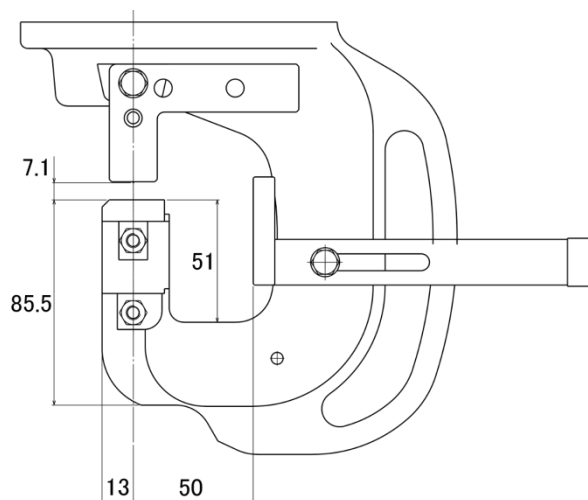
ダイスアダプター使用時
