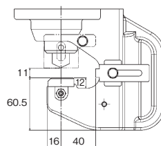
ハウジング寸法図
