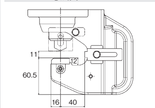
ハウジング寸法図
