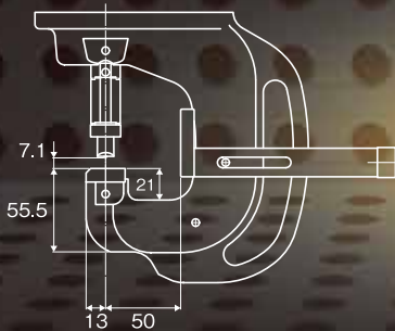
寸法図
